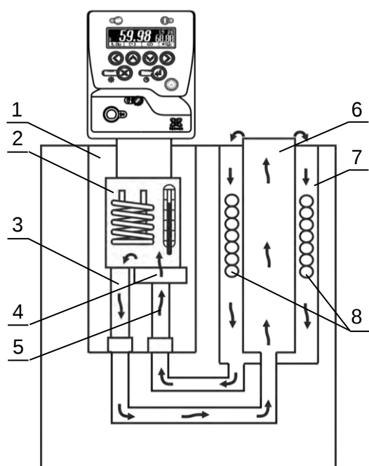
Рисунок 2 — Устройство термостата
